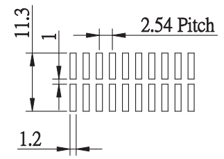
P.C.Board Layout
